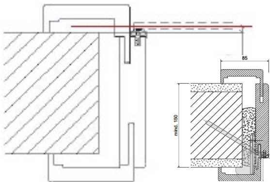
Ościeżnica regulowana drewniana warianty mocowania
