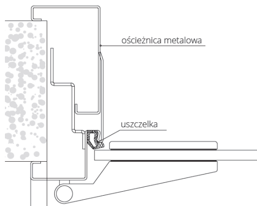
Ościeżnica metalowa regulowana
